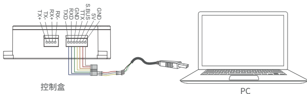
接线图
